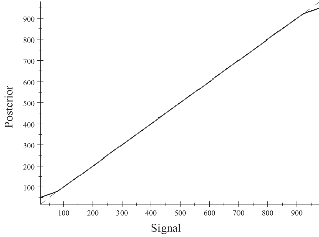
Figure A.2 Turn one posterior
